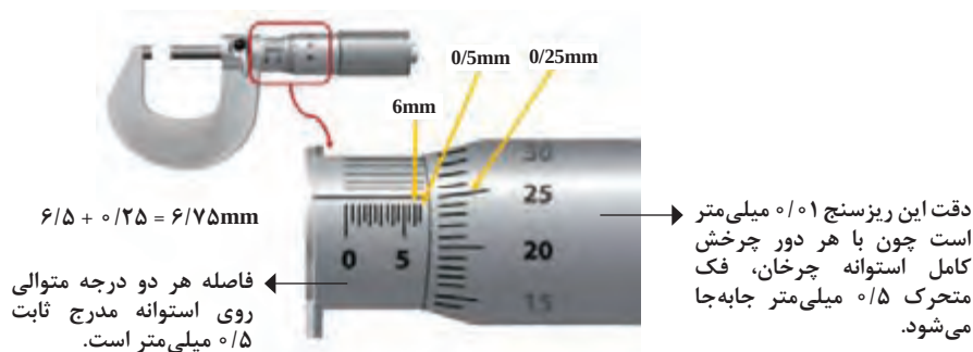
شکل ۱۴-۱ نحوه خواندن نتیجه اندازه‌گیری با ریزسنج ۰/۰۱ میلی‌متری
