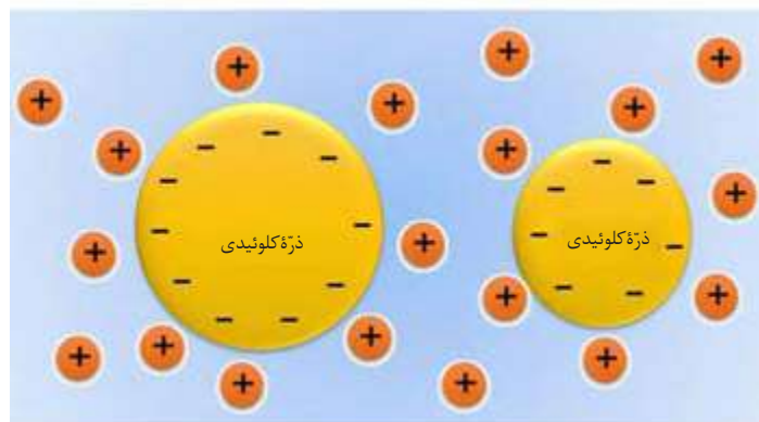
شکل ۱۰. ذره‌های کلئیدی
